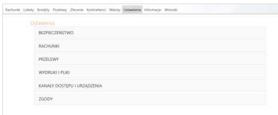
Rys. 43 Okno „Ustawienia”
